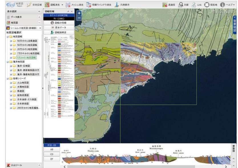
いろいろな地質図
